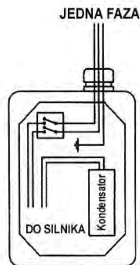
Schemat skrzynki elektrycznej
