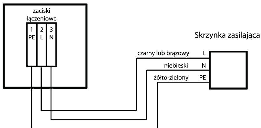
Schemat połączenia elektrycznego urządzenia z rozdzielnią główną w układzie zasilania TN-S
